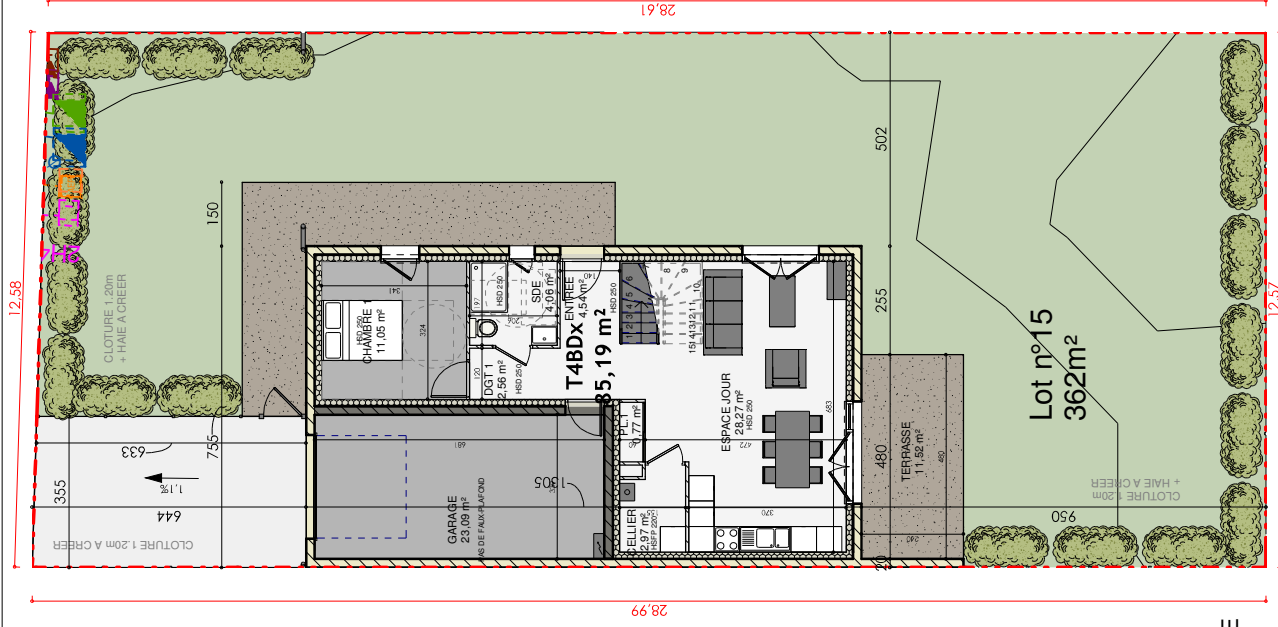
PLAN DE MASSE 1 : 125
