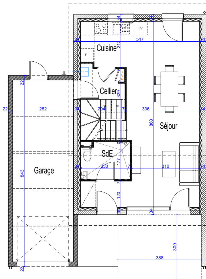
Vue en plan du logement RdC
