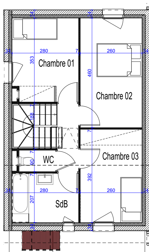
Vue en plan du logement Etage
