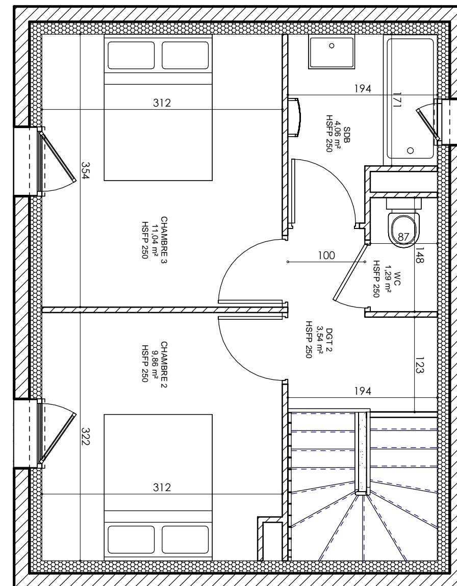
Plan Etage - 1/50
